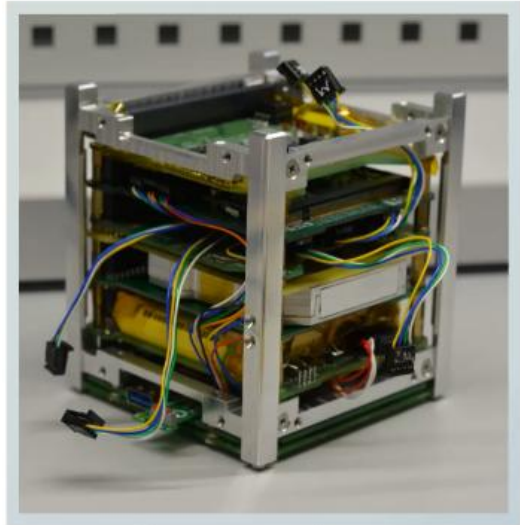
Сборка CubeSat
