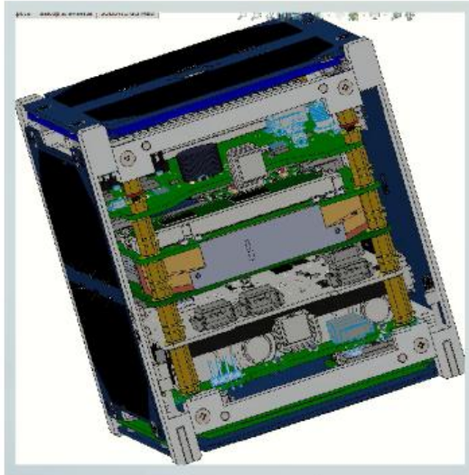
3D-модель CubeSat в программе SolidWorks
